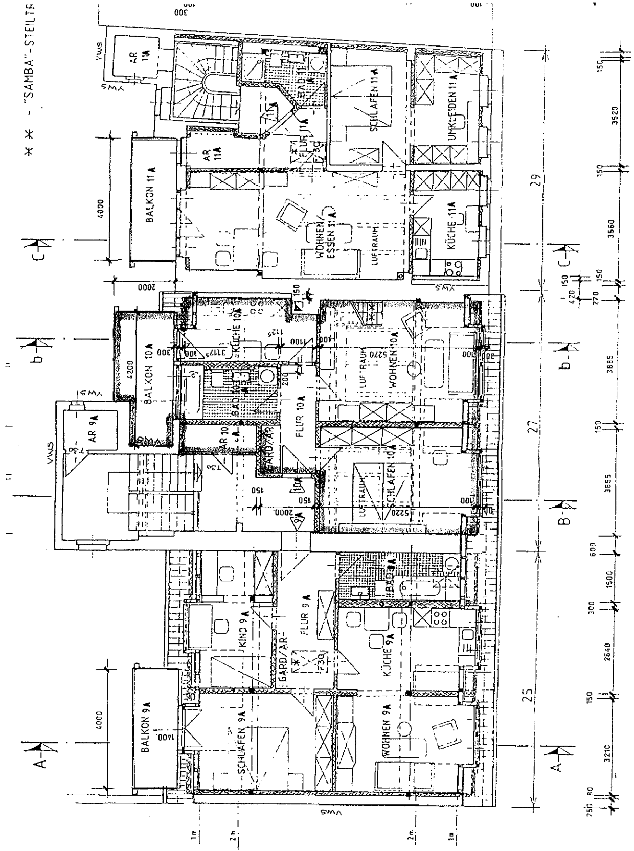
Grundriss Dachgeschoss
